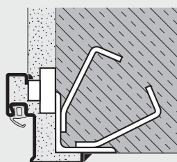
Rohová zárubeň Svařovaná montáž
