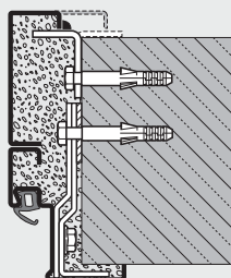
Rohová a přídatná zárubeň Zakrytá hmoždinková montáž
