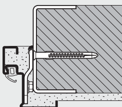
Rohová zárubeň Svařovaná montáž
