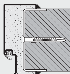
Obvodová zárubeň B73 Svařovaná montáž
