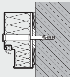
Bloková zárubeň Skrytá hmoždinková montáž
