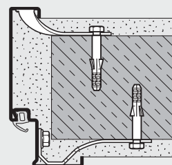
Obvodová zárubeň Montáž pomocí hmoždinkových kotev do zdiva
