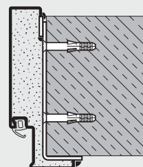
Obvodová zárubeň Svařovaná montáž
