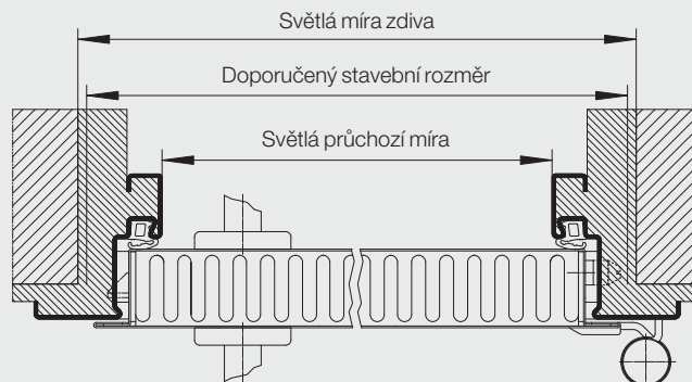
Vodorovný řez jednokřídlými dveřmi
