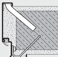
Obvodová zárubeň Montáž s kotvami do zdiva
