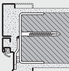
Rohová a doplňková zárubeň Svařovaná montáž
