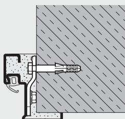
Rohová zárubeň Hmoždinková montáž
