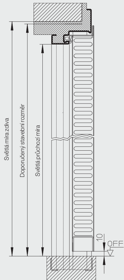
Svislý řez
