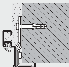
Rohová zárubeň Montáž ve stěně
