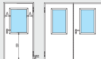
Provedení prosklení 2
