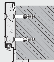
Obvodová zárubeň hmoždinková montáž skrz ostění
