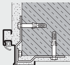
Rohová zárubeň Montáž pomocí hmoždinkových kotev do zdiva
