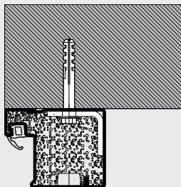
Bloková zárubeň skrytá montáž pomocí hmoždinek
