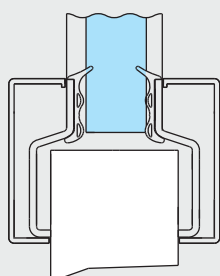
Hliníkový krycí profil
