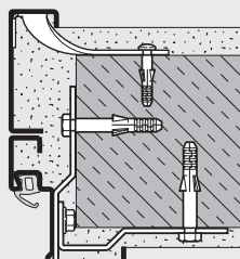
Rohová zárubeň s přídatnou zárubní Montáž pomocí hmoždinkových kotev do zdiva
