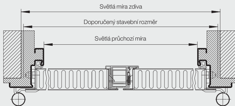
Vodorovný řez dvoukřídlými dveřmi
