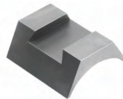
Hülsekopfsattel für Repetierbüchsen. Länge: 38 mm, BH: 6,0 mm
