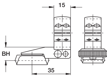
Klemmringsen aus Aluminium \varnothing 1\frac{1}{2} mm Verlängerung: 35 mm
