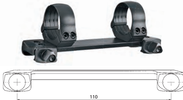
Bolzenabstand 110 mm, Länge 130 mm
