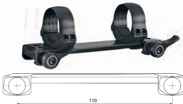
Bolzenabstand 110 mm, Länge 130 mm
